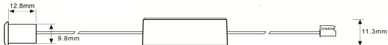
SEITENANSICHT
